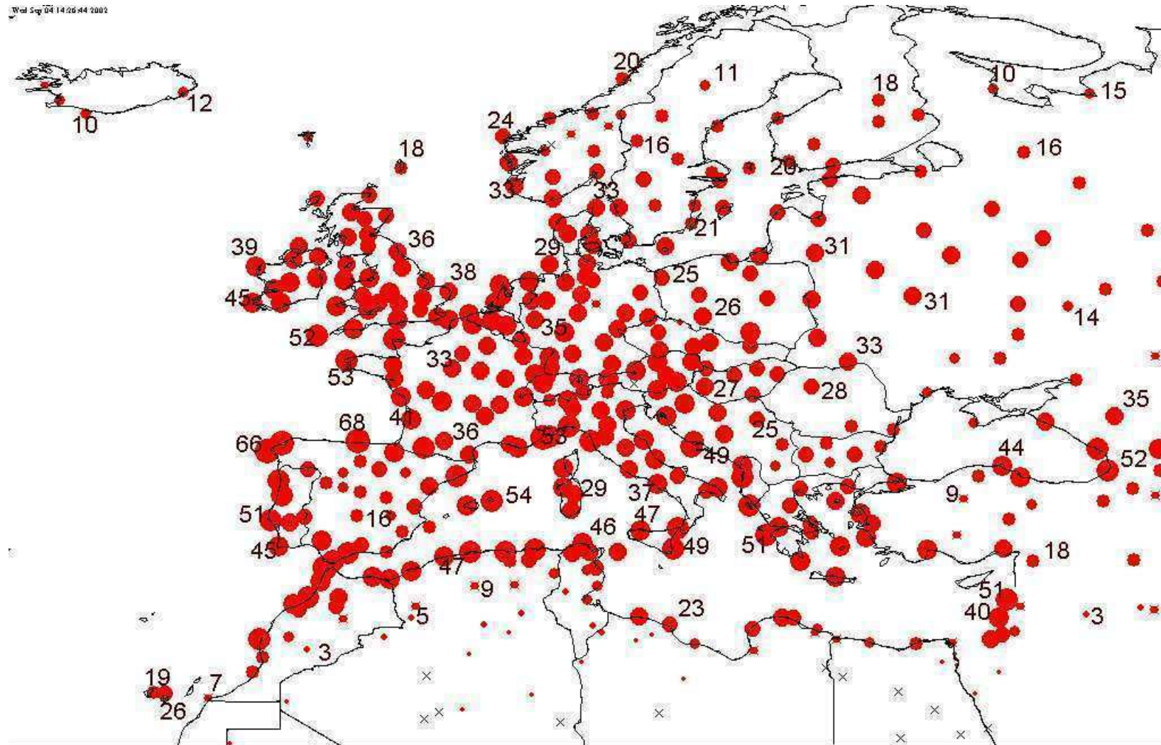
Fig. 3 Tecia solanivora : Indice Eco-climatique dans la zone OEPP
